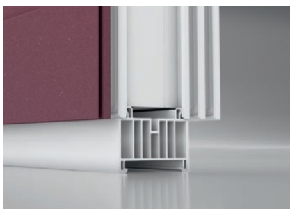
Listwa transportowo-montażowa
