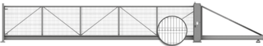
BRAMA PRZESUWNA Z WYPEŁNIENIEM W POSTACI PANELI KRATOWYCH VEGA B PRZYKRĘCONYCH DO KONSTRUKCJI - WIDOK OD STRONY POSESJI.
